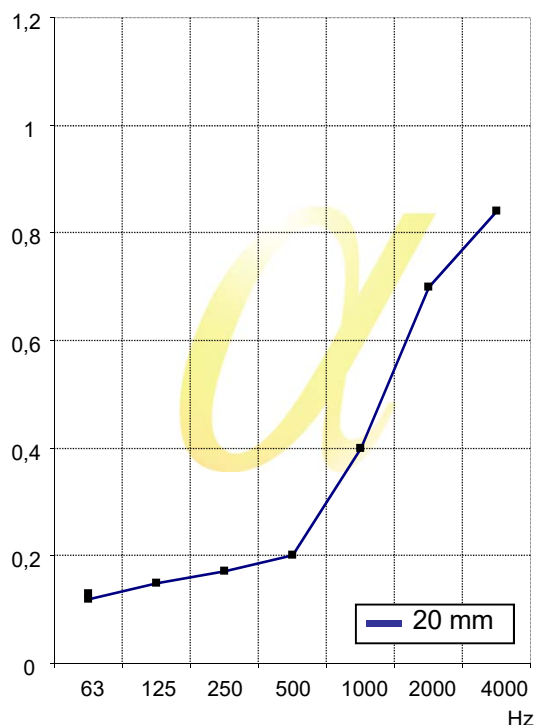
Coefficiente de absorción acústica Sabine, \alpha_s .
